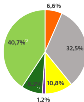
Bundesdeutscher Strommix
